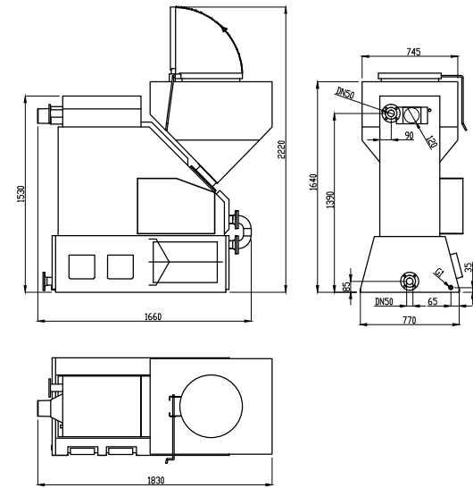
kotel EKOEFK 48(4) Horni bez serva-250l
