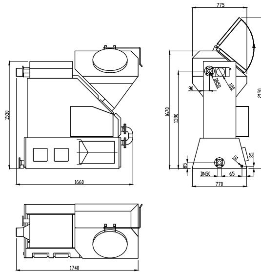
kotel EKOEFK 48(4) Bocni bez serva-250l
