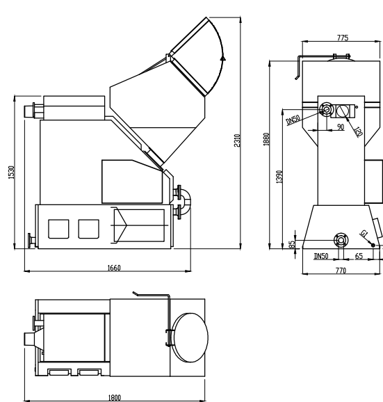
kotel EKOEFK 48 (4) Celni Zv.-bez serva-360l
