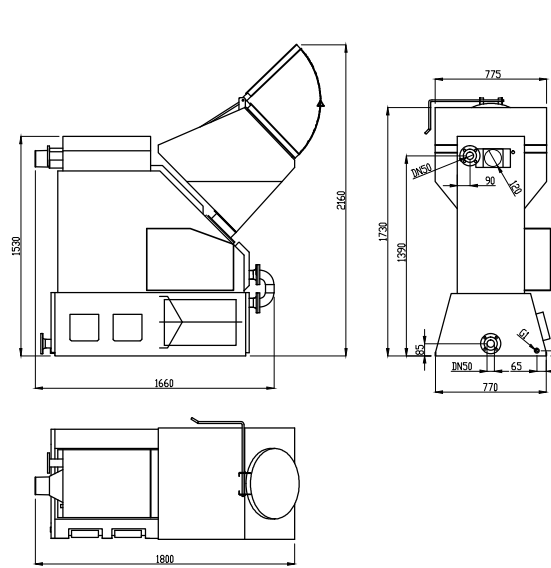
kotel EKOEFK 48(4) Celni bez serva-250l
