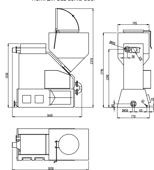
kotel EKOEFK 48 (4) Horni Zv.-bez serva-360l
