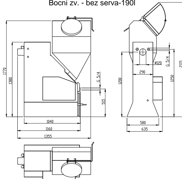
kotel Ekoefekt 24(4) Bocni zv. - bez serva-190I
