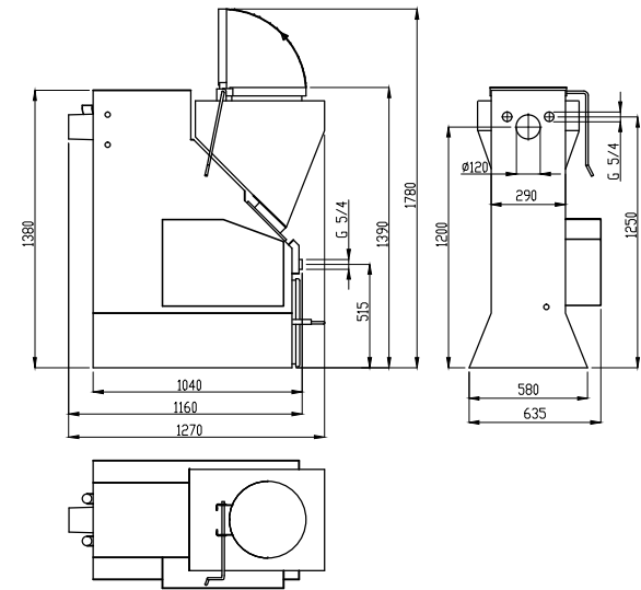
kotel Ekoefekt 24(4) Horni - bez serva -150I
