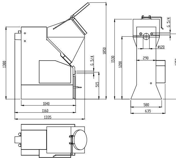
kotel Ekoefekt 24(4) Celni zv. - bez serva -180I
