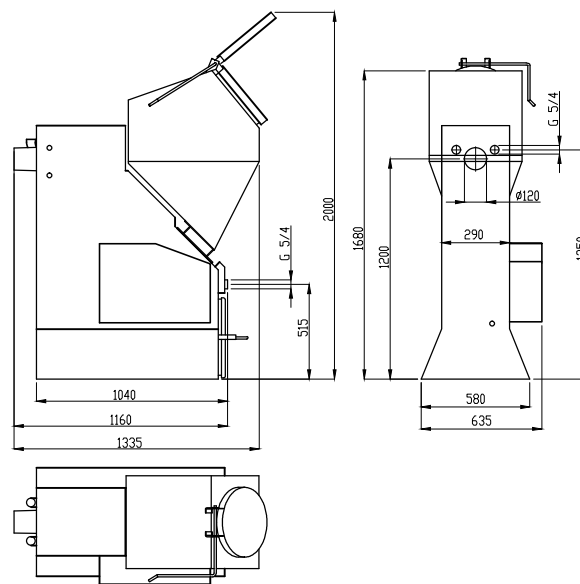
kotel Ekoefekt 24(4) Celni zv. - bez serva -180I
