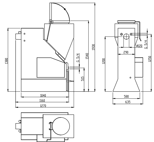
kotel Ekoefekt 24(4) Horni zv. - bez serva -180I
