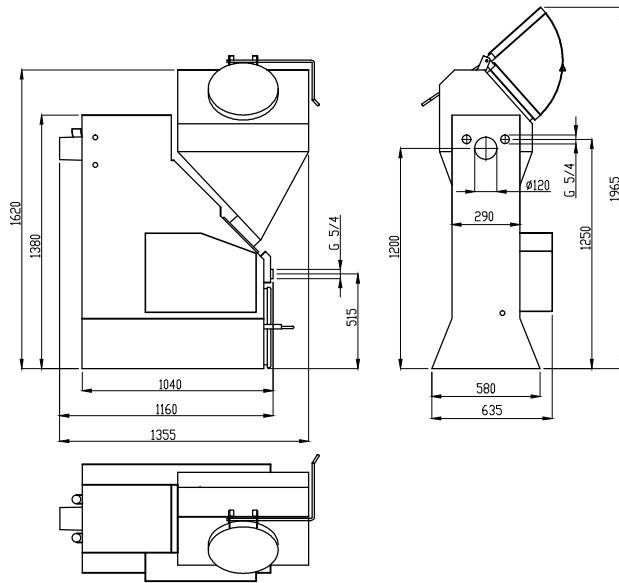
kotel Ekoefekt 24(4) Bocni - bez serva-150I
